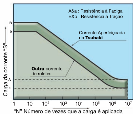
Curva S-N
